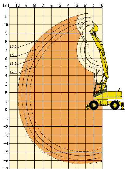
Verstellausleger V5.3
